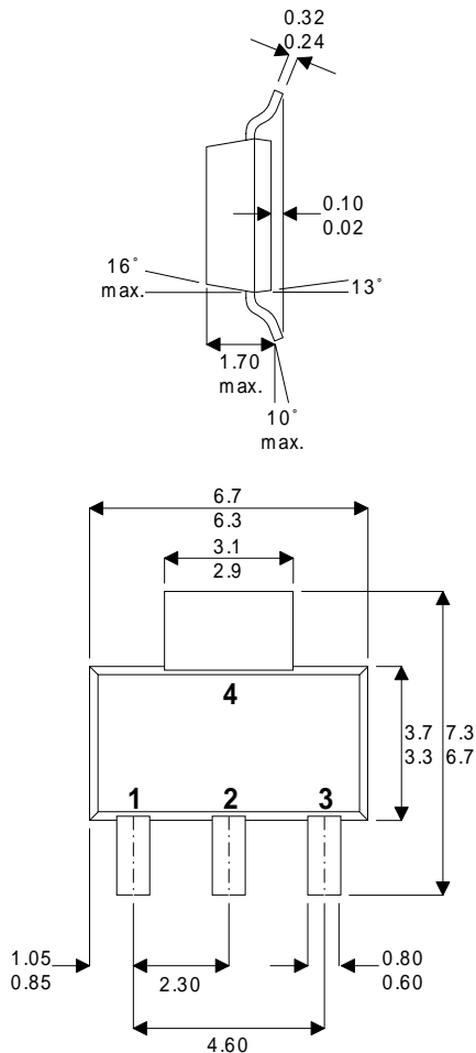
SOT-223
