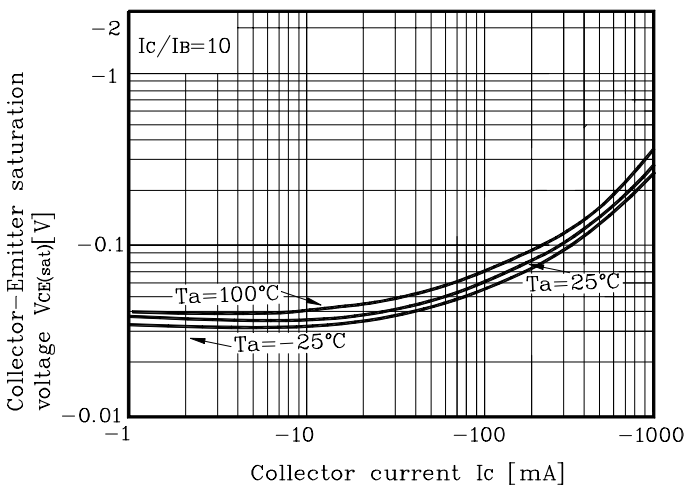
Fig. 5 V_{CE(sat)} - I_C
