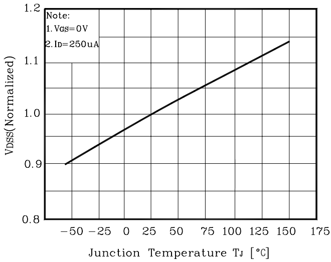
Fig. 7 V_{DS} - T_J
