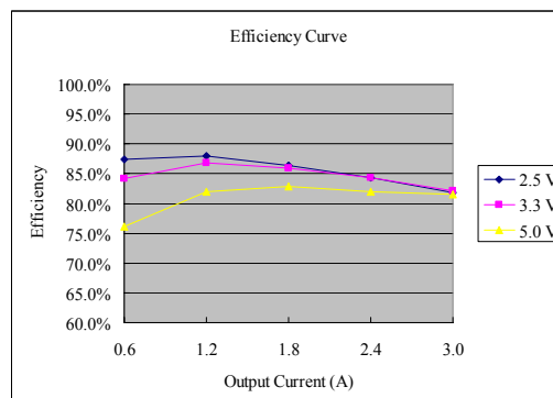
Vo=0.75 V
