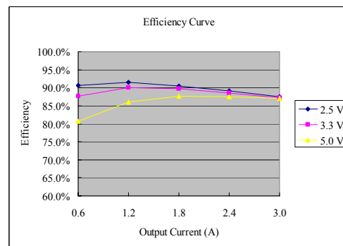
Vo=1.2 V
