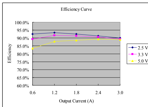
Vo=1.5 V
