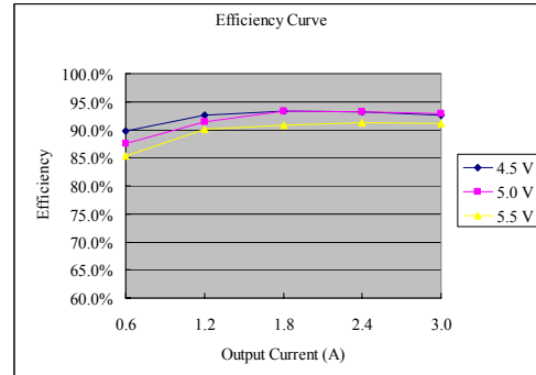
Vo=2.5 V
