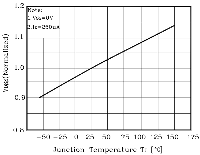
Fig. 7 V_{DSS} - T_J
