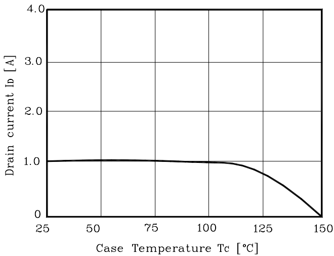
Fig. 9 I_D - T_C
