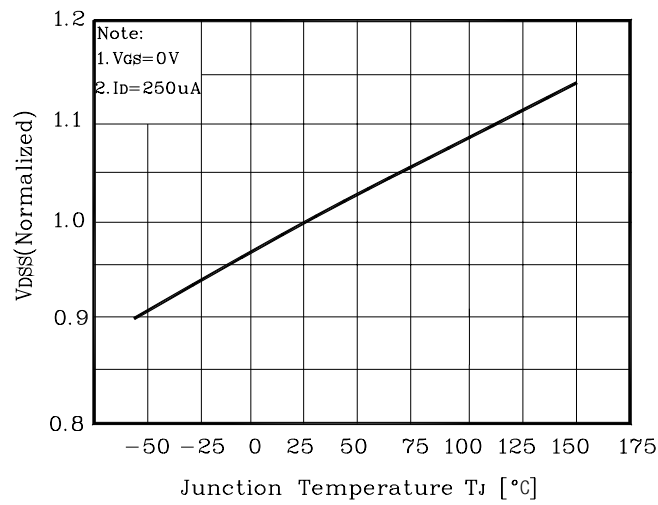
Fig. 7 V_{DS} - T_J
