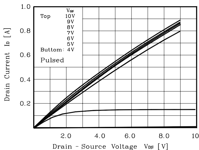
Fig. 1 I_D - V_{DS}
