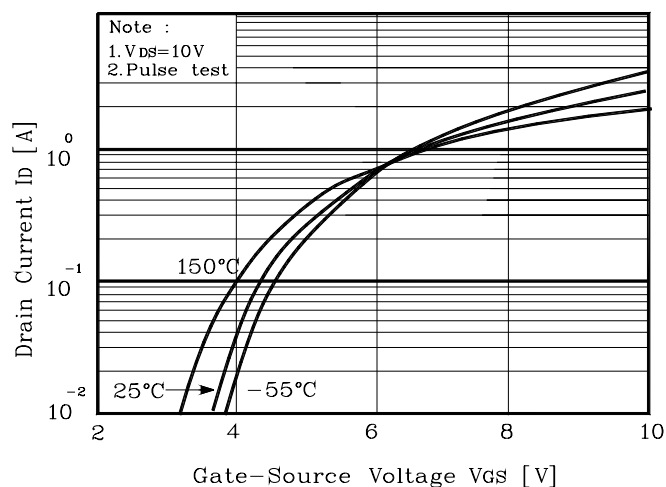
Fig. 2 I_D - V_{GS}
