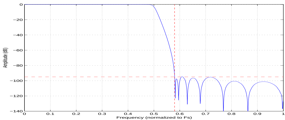
Figure 21. SSM Stopband
