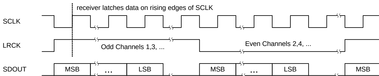
Figure 12. LJ Format
