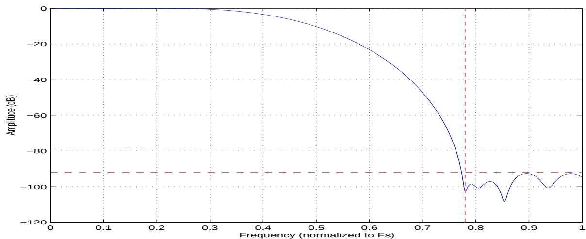
Figure 23. QSM Stopband
