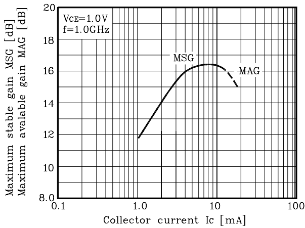
Fig. 12 MSG, MAG-I c
