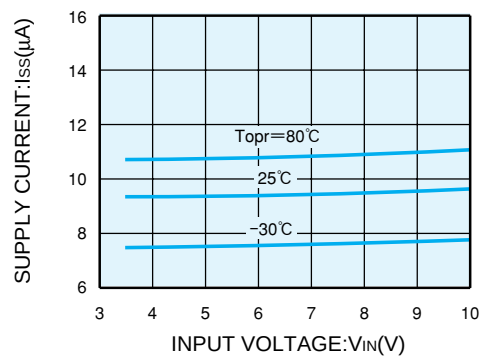
XC62GR3012(3V)
