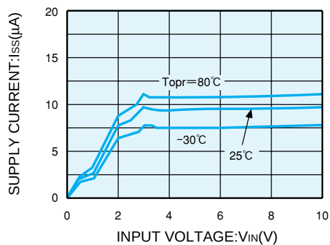
XC62GR3012(3V)
