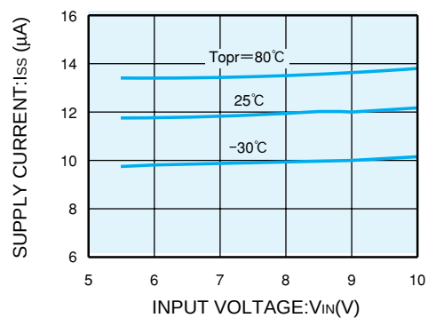
XC62GR5012(5V)
