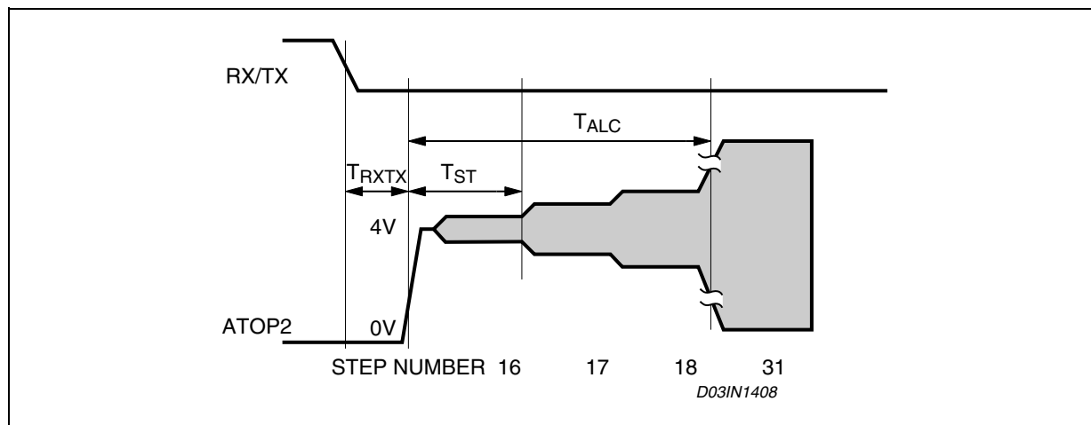
Figure 18. PLI Startup Timing Diagram
