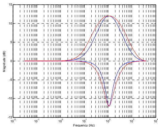
Figure 48 EQ Band 3 – EQ3BW=0, EQ3BW=1
