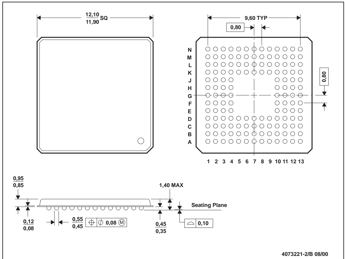
GGU (S-PBGA-N144)
