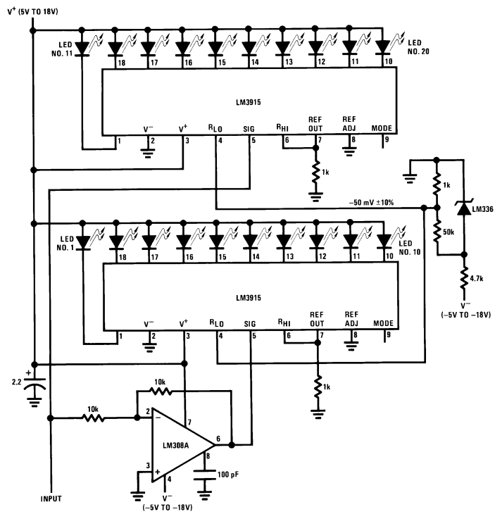
Precision Null Meter
