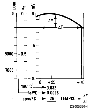
LM385
