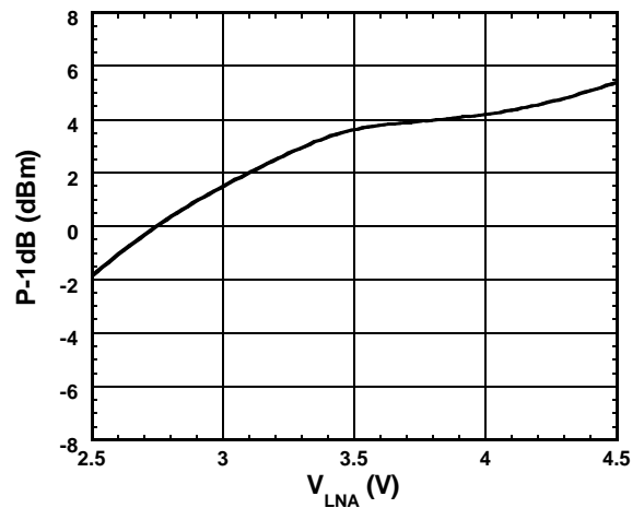
P-1dB vs. V_{LNA} ( f=1900MHz )
