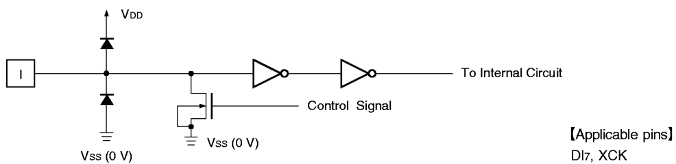
Fig. 2 Input Circuit (2)
