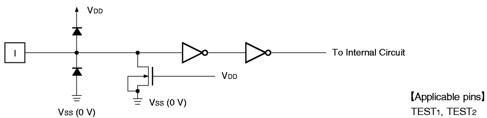
Fig. 3 Input Circuit (3)
