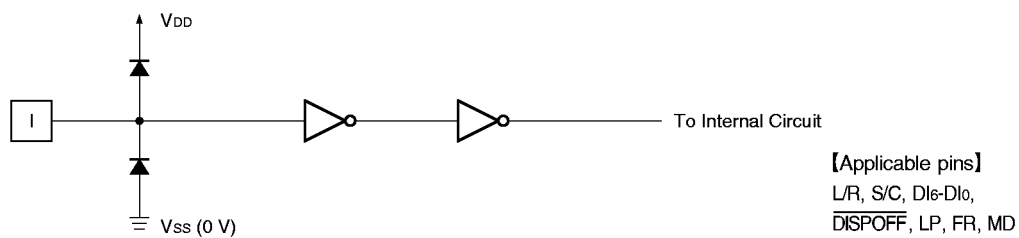
Fig. 1 Input Circuit (1)
