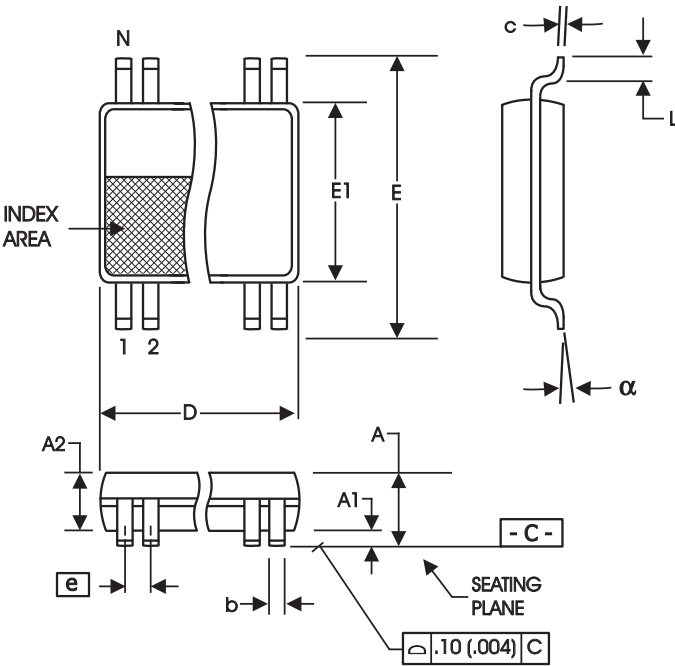
209 mil SSOP
