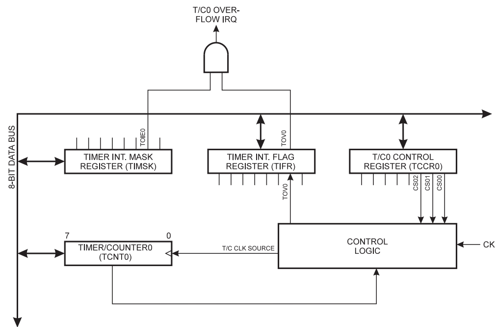
Figure 33. T/C0 方框图
