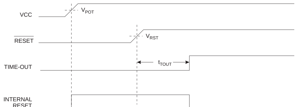
Figure 22. 外部控制 MCU 启动 \overline{RESET}
