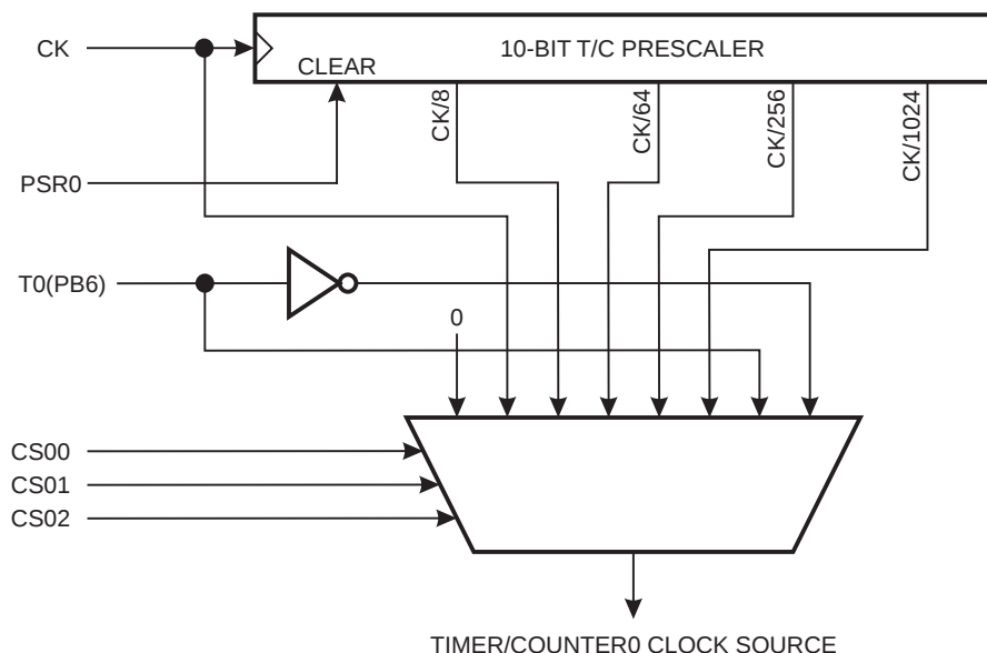
Figure 31. T/C0 预分频器
