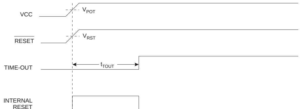
Figure 21. 通过 VCC, MCU 启动 \overline{RESET}
