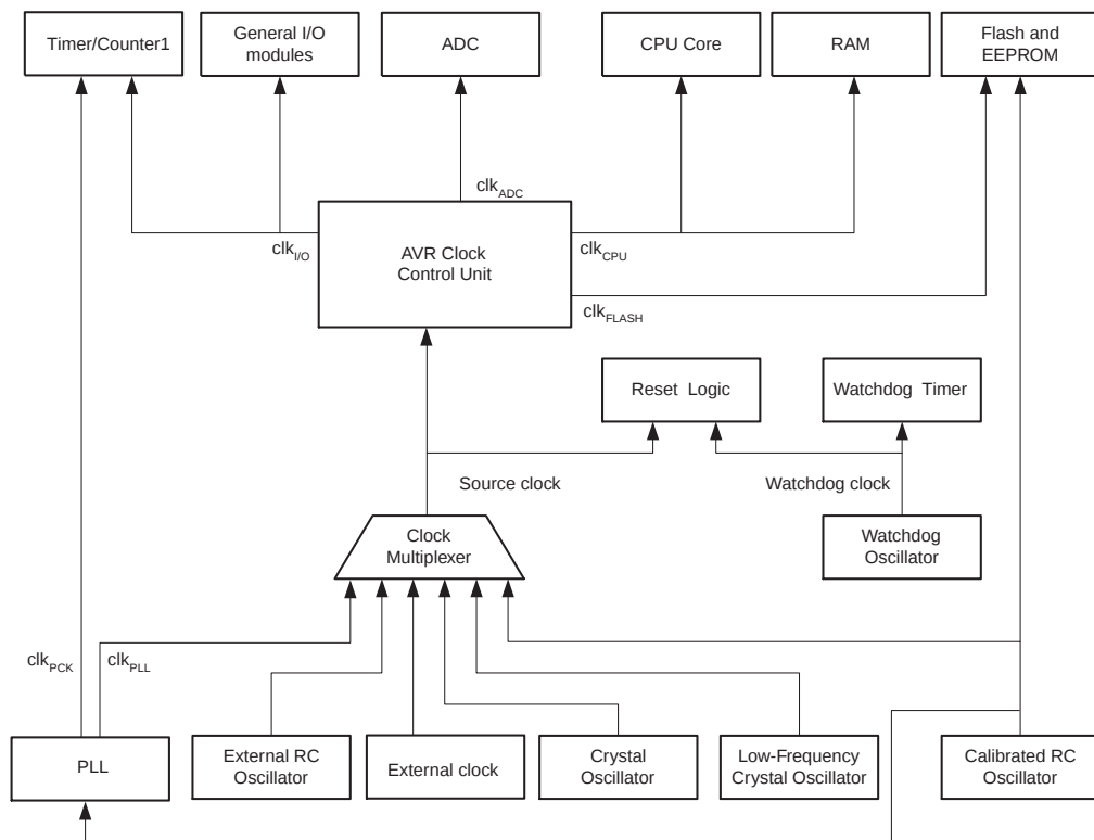
Figure 26. 时钟分布
