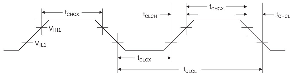
Figure 70. 外部时钟驱动波形
