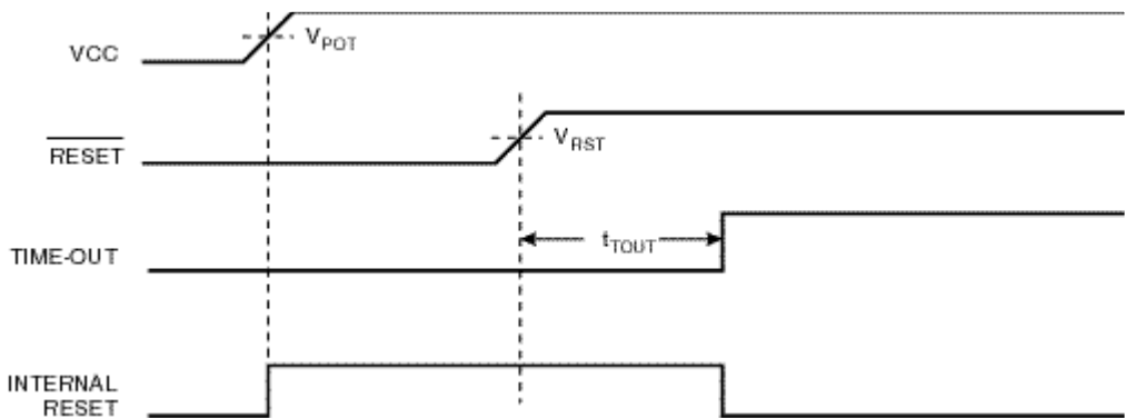
图 26 MCU 启动，/RESET 由外电路控制
