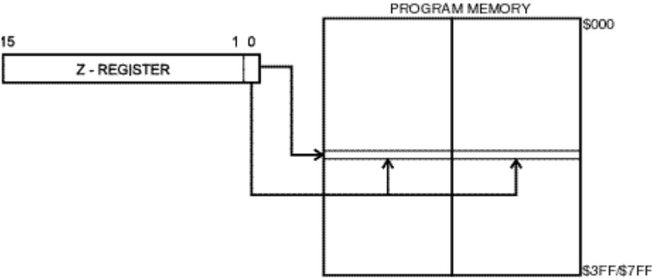
间接程序寻址，JUMP 和 ICALL 图 19
