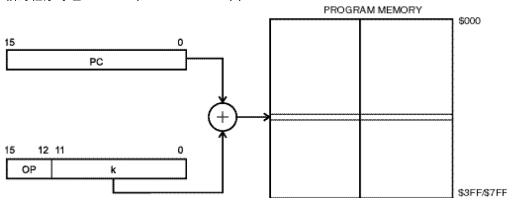
相对程序寻址，RJMP 和 RCALL 图 20
