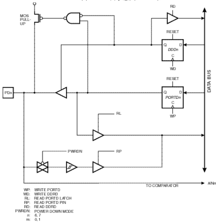
图 61 D 口示意图 (PD6 和 PD7)
