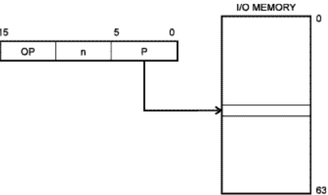
I/O 直接寻址 图 12
