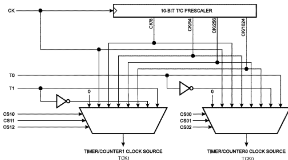
图 30 T/C1 和 T/C0 的预分频器
