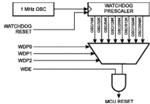
图 35 看门狗定时器
