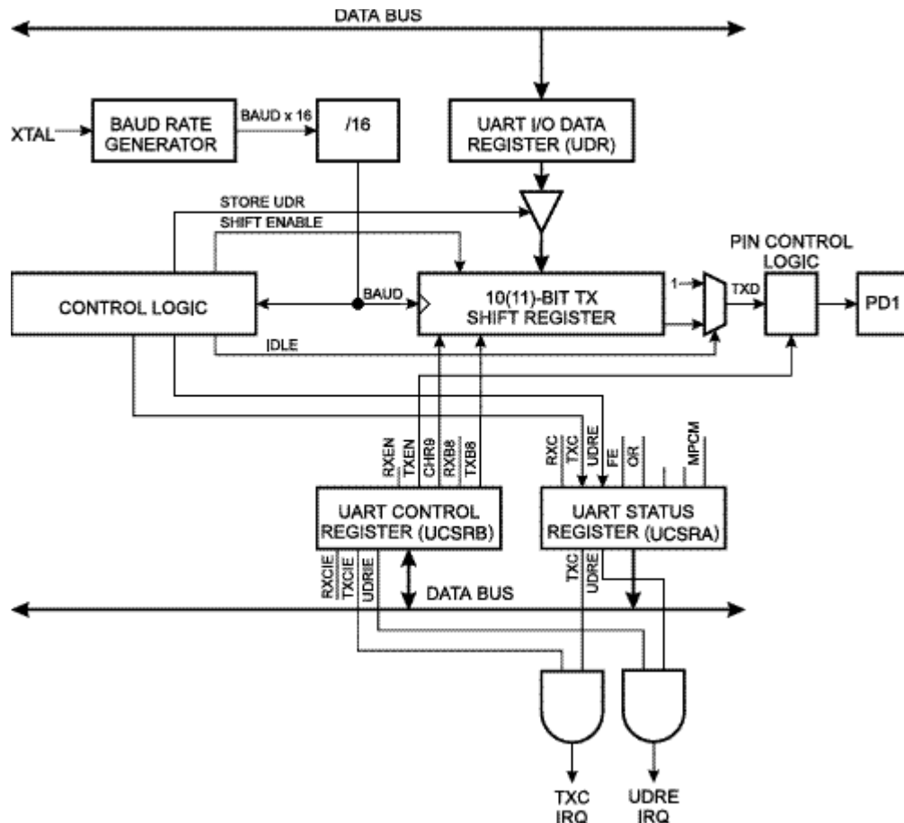
图 40 UART 发送器
