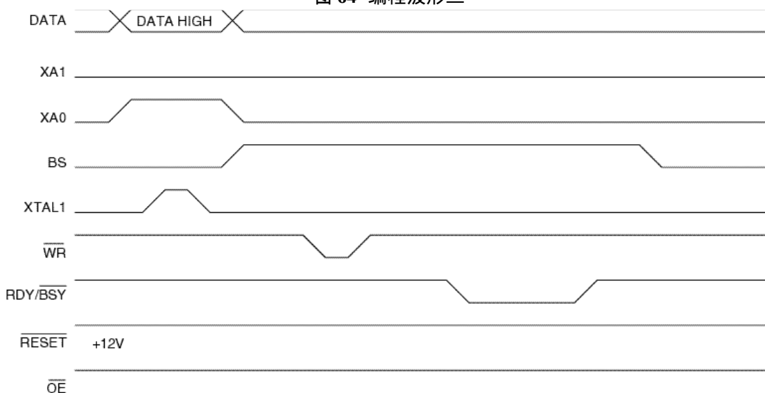
图 64 编程波形二
