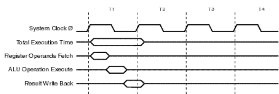
图 22 单时钟 ALU 操作
