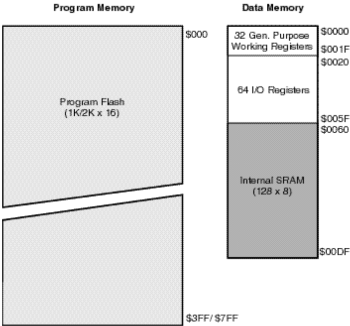
图 6 内存映像
