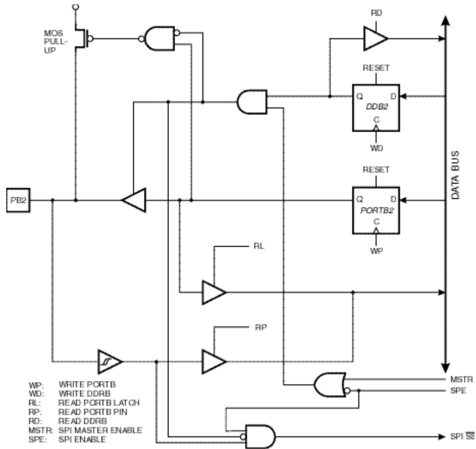
图 52 B 口示意图 (PB2)
