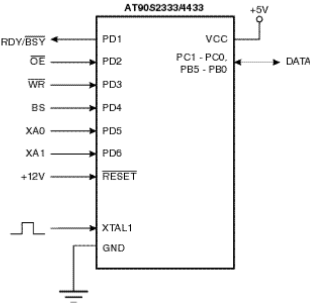
图 62 并行编程
