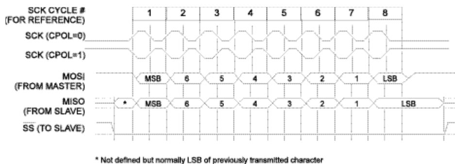
图 39 SPI 传输格式 (CPHA=1, DORD=0)
