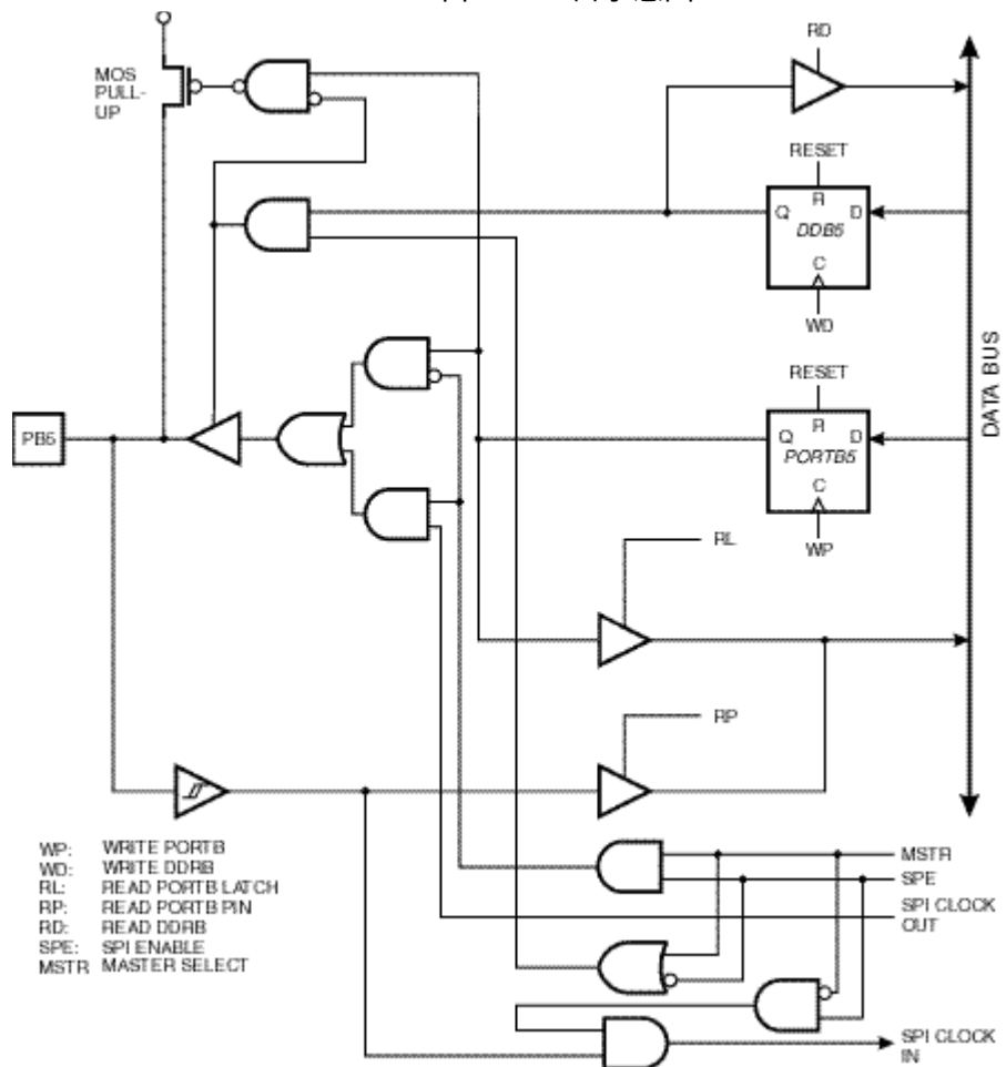
图 55 B 口示意图 (PB5)
