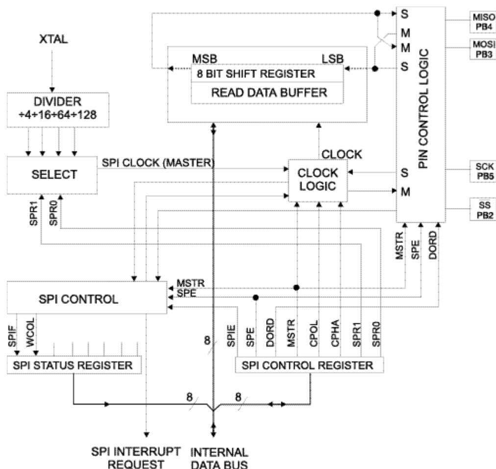
图 36 SPI 方框图
