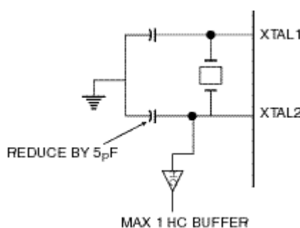
图 3 利用 MCU 振荡器作为外围器件的时钟
