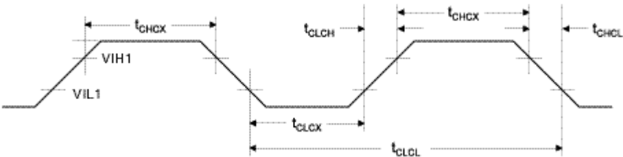
图 69 外部时钟
