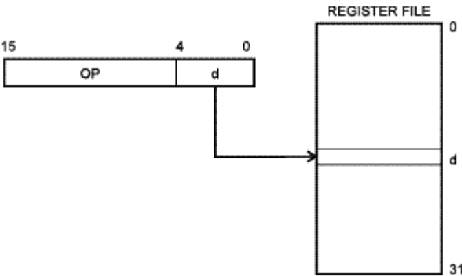
双寄存器直接寻址 图 11
