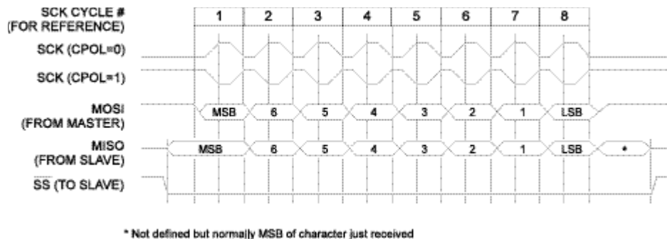
图 38 SPI 传输格式 (CPHA=0, DORD=0)
