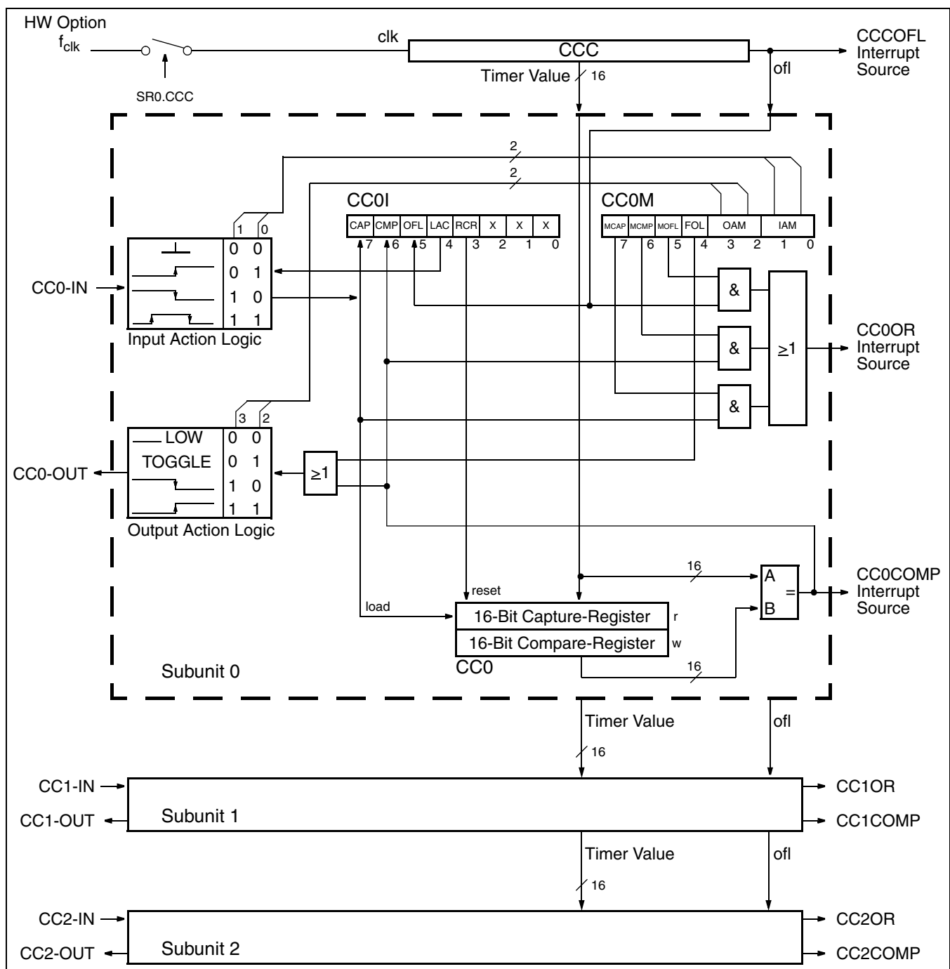
Fig. 15-1: CAPCOM Module Block Diagram
