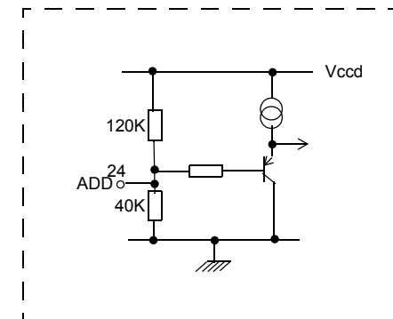
ADD input
