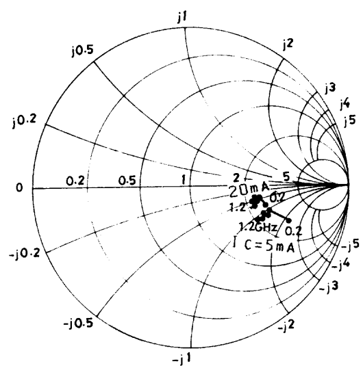
S22e : VCE=10V
