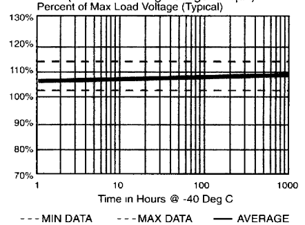
54) Ton Stability
