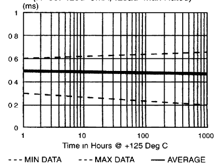
60) Toff Stability
