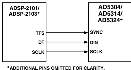
Figure 10. AD5304/AD5314/AD5324 to ADSP-2101/ADSP-2103 Interface
