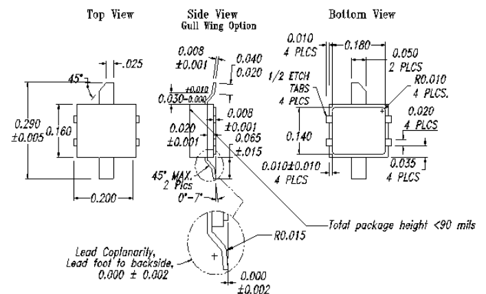
Polyfet S02 Package
