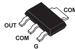
SOT-223 ACS108-5SN
