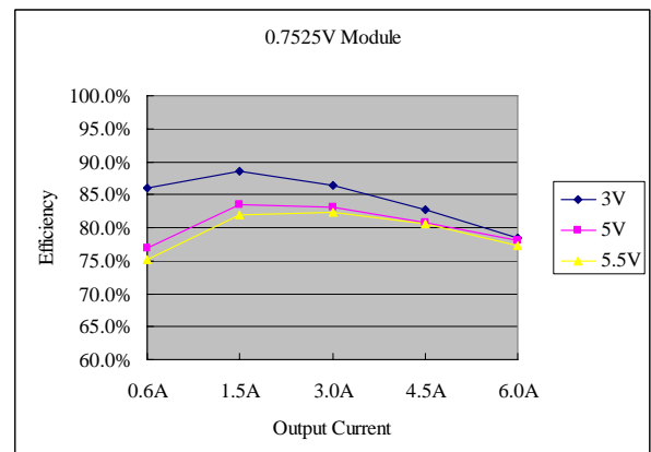
Vo=0.7525 V
