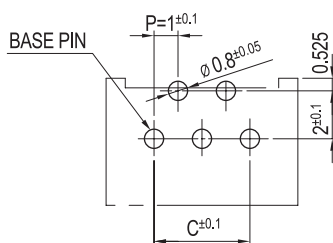
P.C.B. LAY-OUT(A-TYPE)
