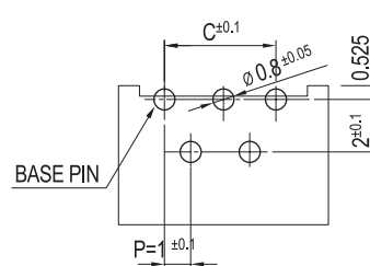
P.C.B. LAY-OUT(B-TYPE)
