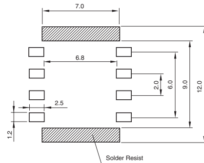
LAND PATTERNS(mm) 推奨ランド寸法
