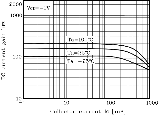
Fig. 4 h_{FE} - I_C
