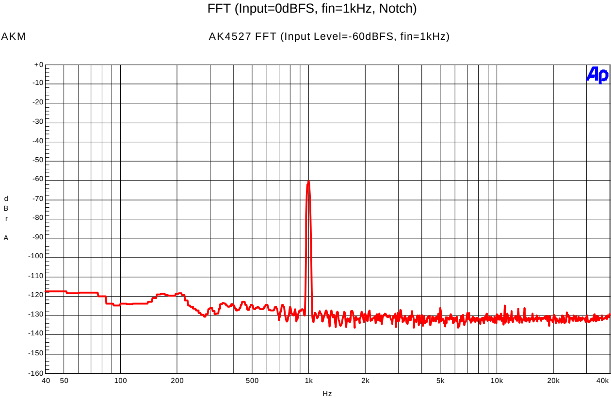
FFT (Input=-60dBFS,fin=1kHz)
