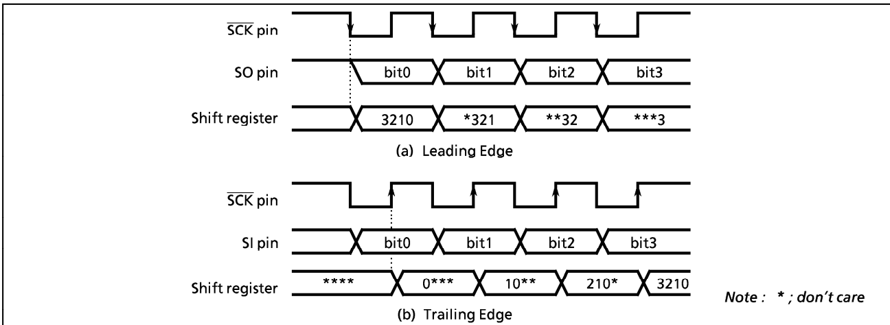
Figure 2-40. Shift Edge
