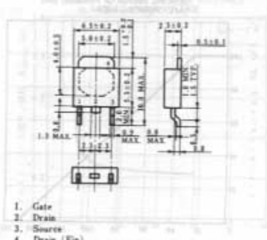
2SJ132-Z外形図
