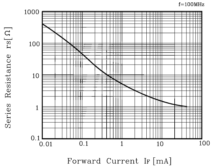
Fig. 2 r_s - I_F
