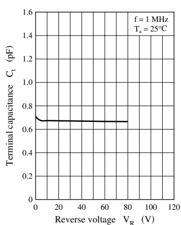
C_t - V_R
