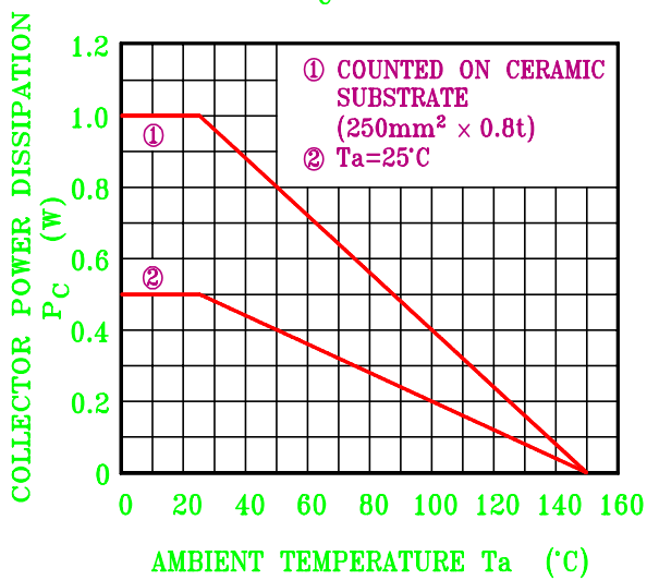
P_C - T_a
