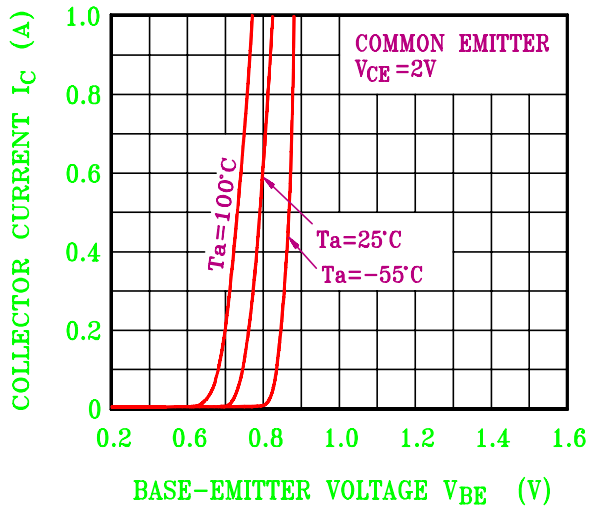
I_C - V_{BE}
