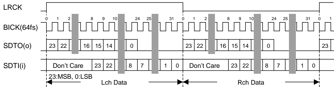
図2. Mode 1 タイミング
