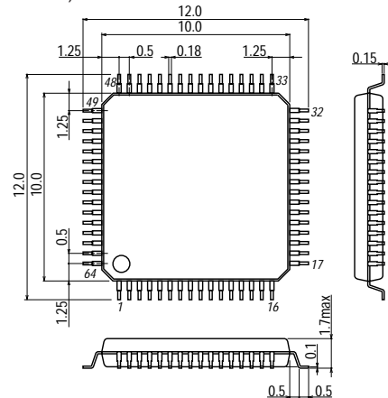
SANYO : SQFP64
