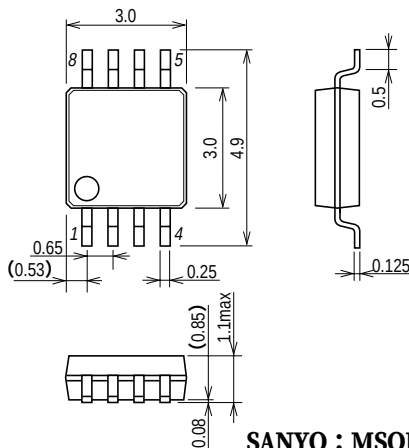
外形図 3245A (unit : mm)
