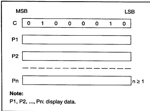
Figure 30. MWRITE parameters
