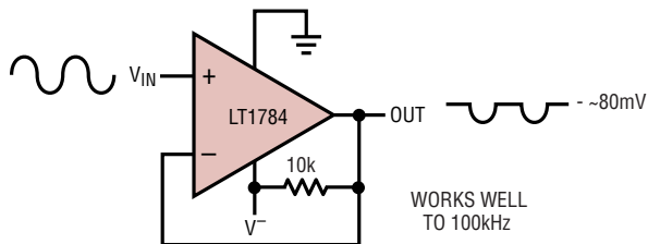
Negative Rectifier
