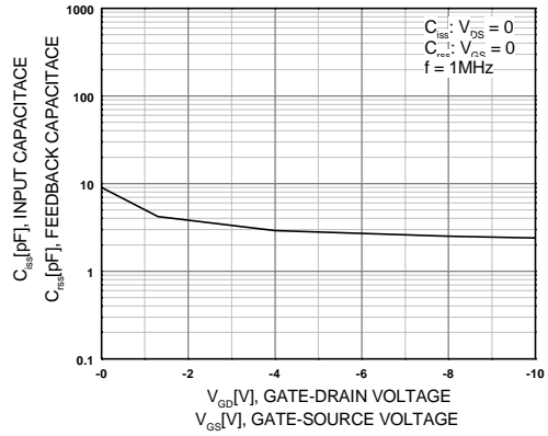
Figure 8. C_{iss}-V_{GS} , C_{rss}-V_{GD}
