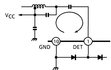
Fig.3 Rectifier Loop
