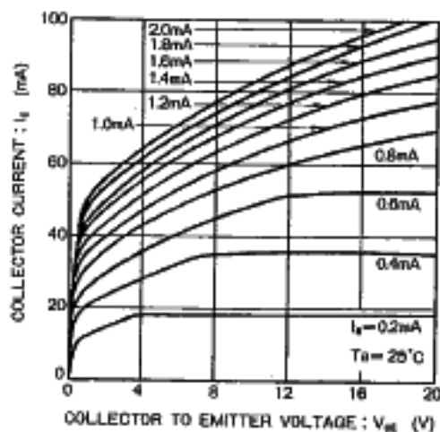
Fig. 4 エミッタ接地出力静特性 (II)
