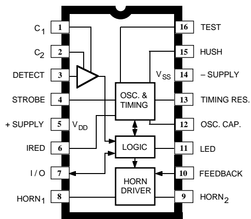
Dwg. PC-007
