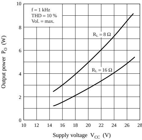
P_O - V_{CC}
