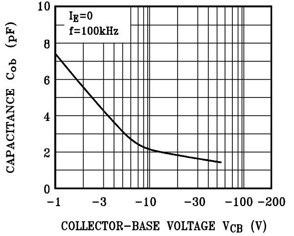
C_{ob} - V_{CB}
