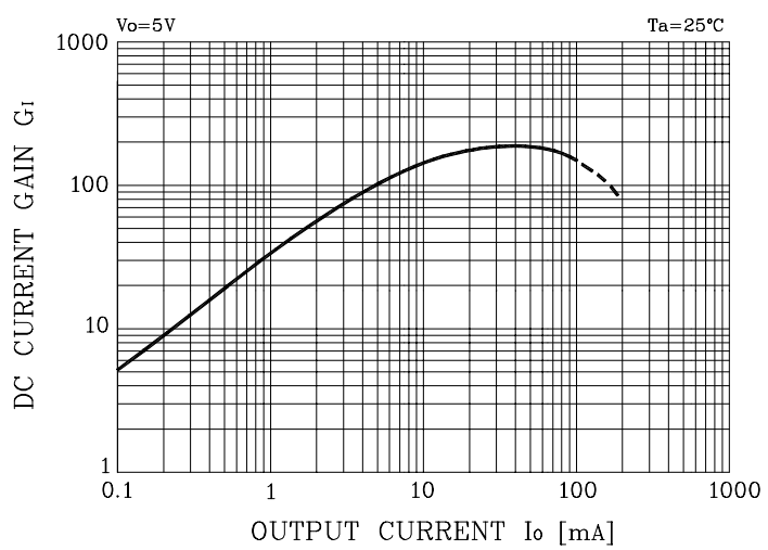
Fig. 3 G_I - I_o
