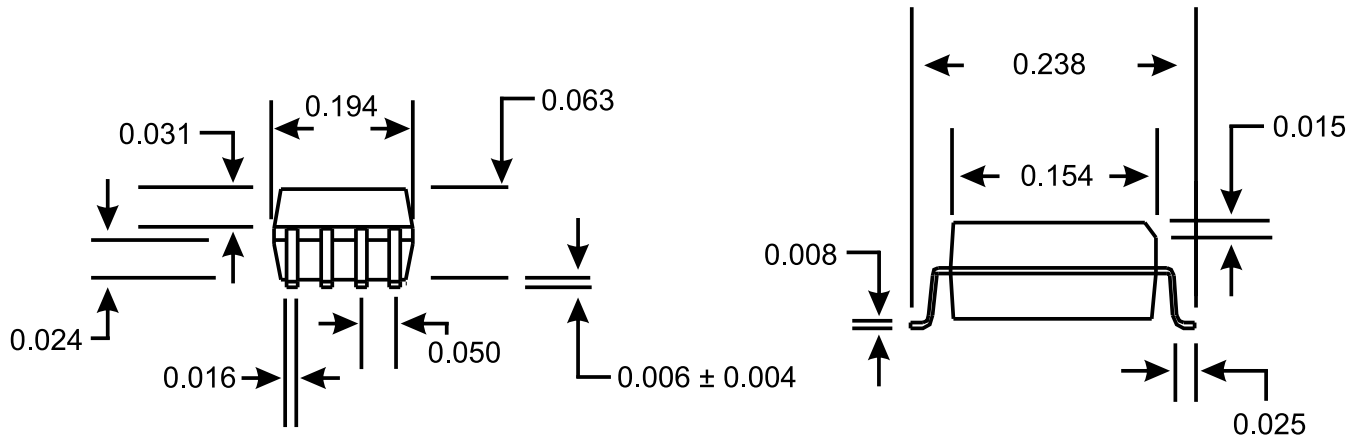
8 - Pin SOIC
