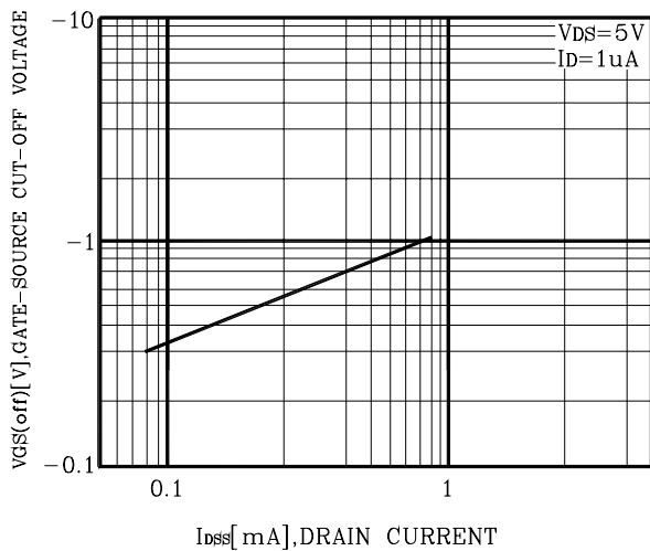
Fig. 5 V_{GS(Off)} - I_{DSS}
